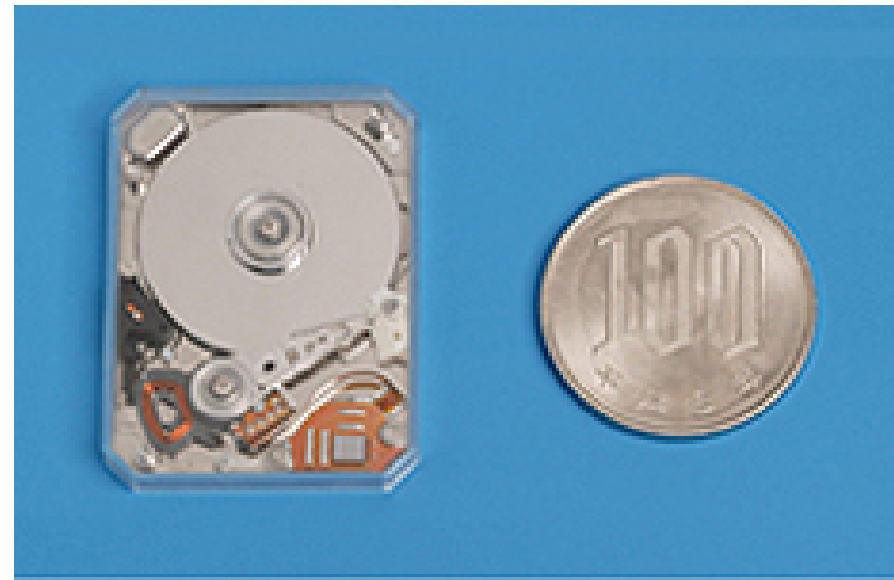
TOSHIBA 東芝「0.85型ハードディスクドライブ」
